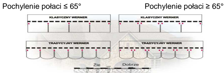
Rys. nr 1. Sposób wbicia gwoźdźcia.
