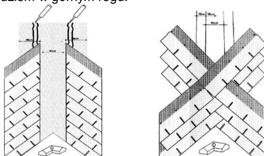
Rys. nr 6. Rysunek kosza otwartego. Rys. nr 7. Rysunek kosza przeplatane.
