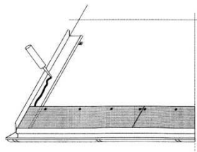
Rys. nr 2. Zastosowanie uszczelniacza dekar skim.
