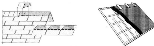
Rys. nr 8. Obróbka kalenic.
