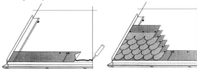
Rys. nr 4. Wykonanie pasa startowego. Rys. nr 5. Rozmieszczenie gontów.
