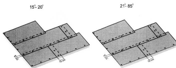
Rys. nr 3. Układanie warstwy podkładowej.
